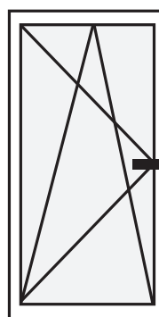
Fenêtre 1 vantail OB1 - Oscillo-battante - Poignée à droite
